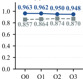
(d) Binutils
